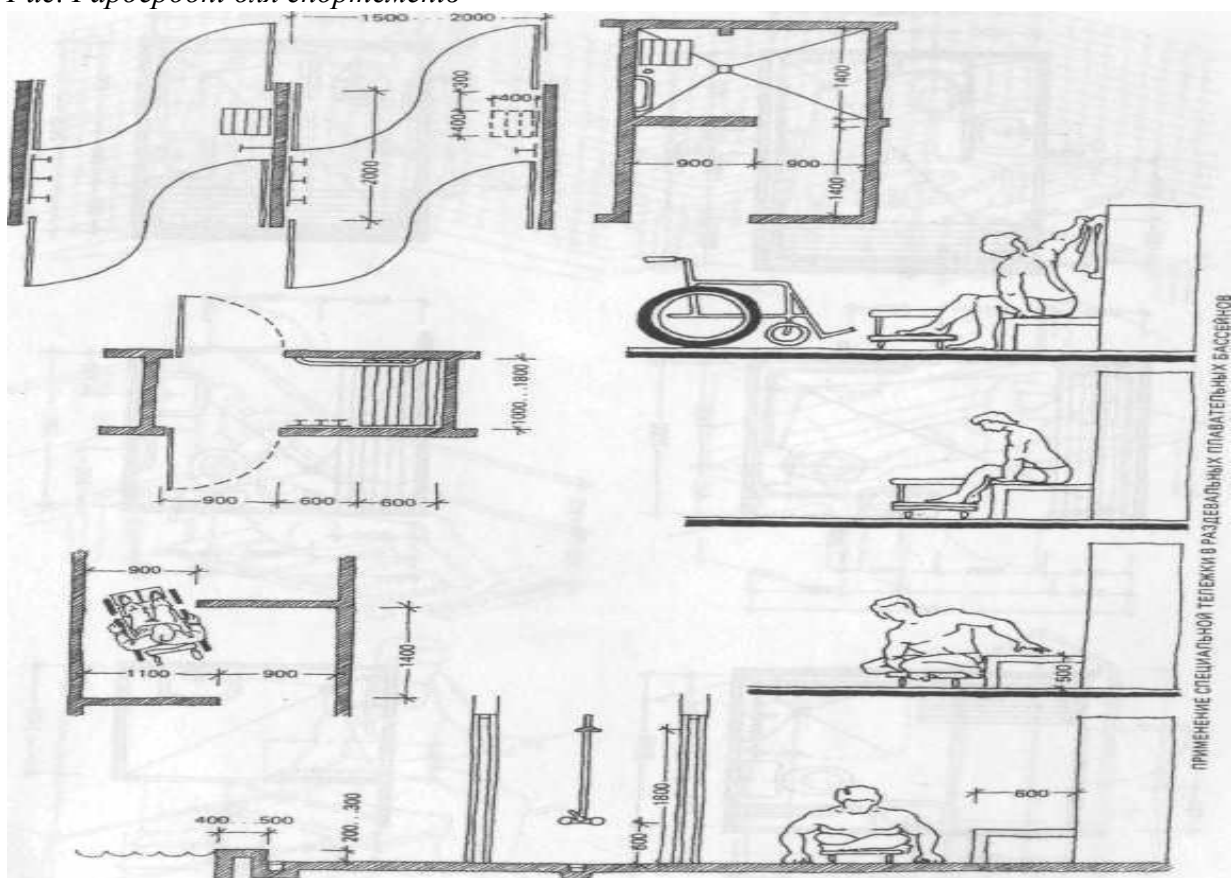
Рис.. Гардеробні для спортсменів (продовження)
